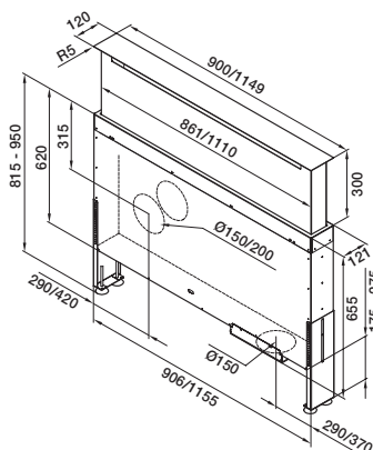
Frontansicht
