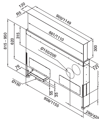
Rückansicht
